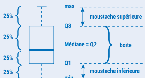
Figure 1 : Schéma de « boîte à moustache » expliquant la répartition de données
